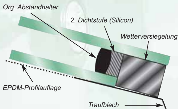
Abb. 3 Fehlerhafte Traufpunktversiegelung
