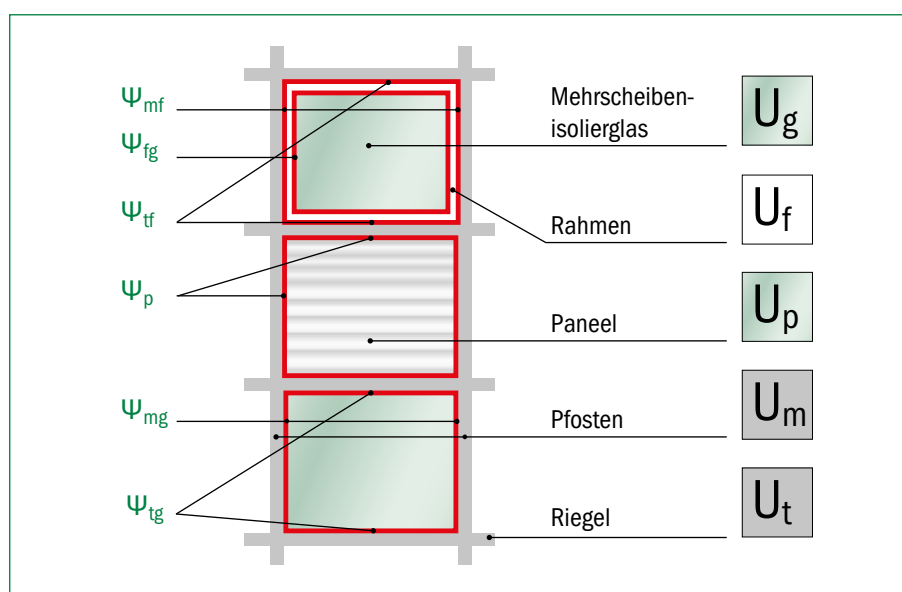
Abb. 14: Musterfassadenelement gemäß EN ISO 12631 [3]
