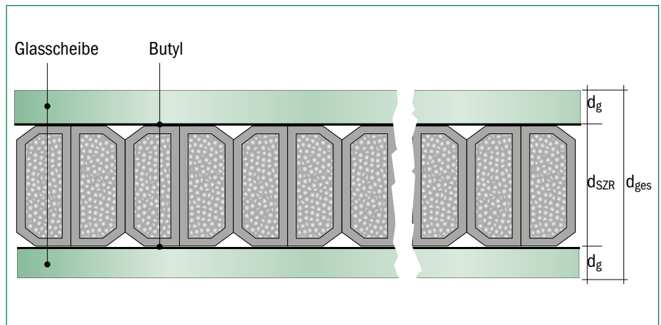
Abb. 7: Aufbau der Probekörper zur Messung der äquivalenten Wärmeleitfähigkeit eines Abstandhalters nach ift-Richtlinie WA 17/1 [5]
