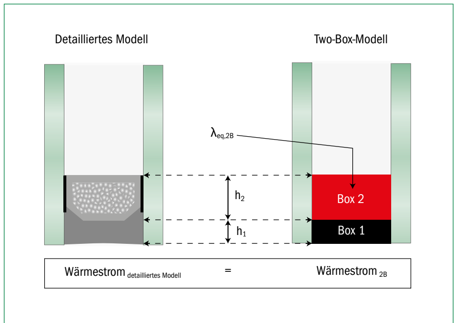
Abb. 8: Schematische Darstellung des Two-Box-Modells
